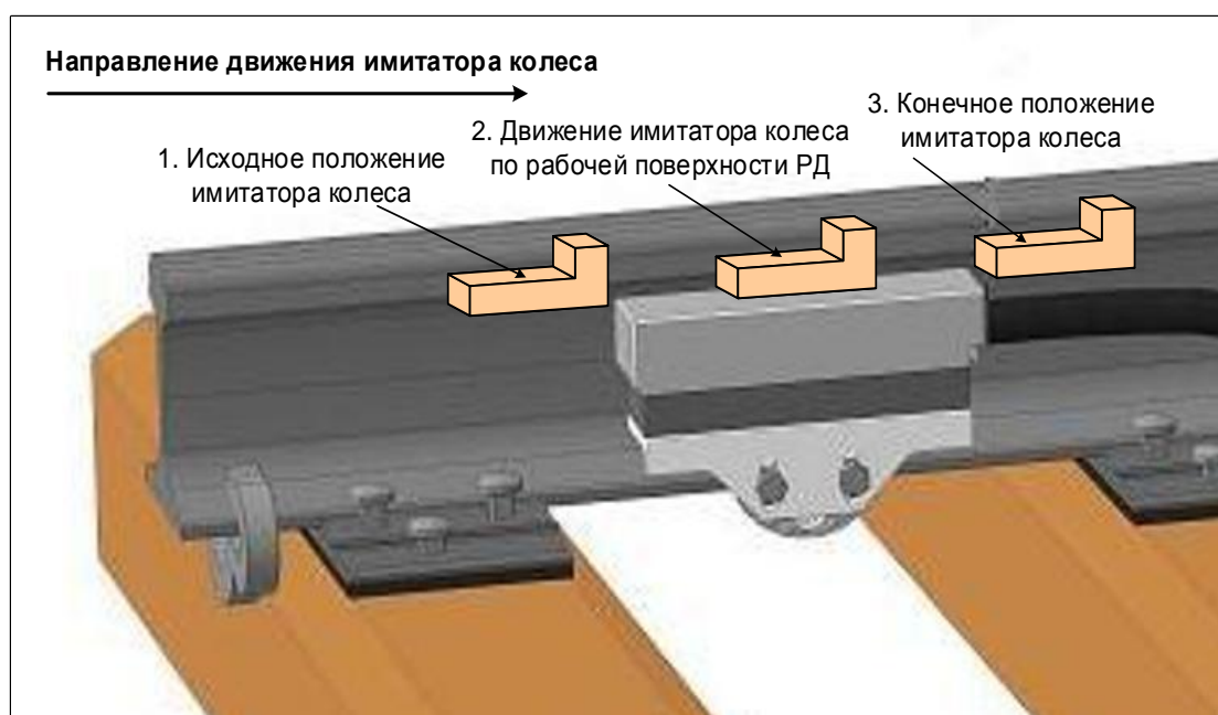
Рисунок 1 – Расположение имитатора колеса относительно датчика
